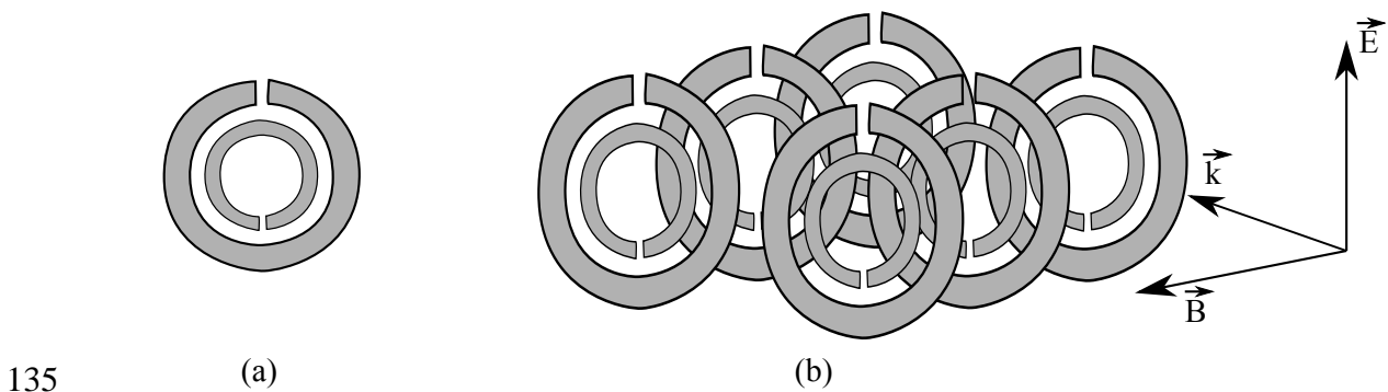
Figure 3 : (a) Principe du résonateur à anneau fendu (split ring resonator SRR) et (b) exemple de réseau périodique de SRR.
