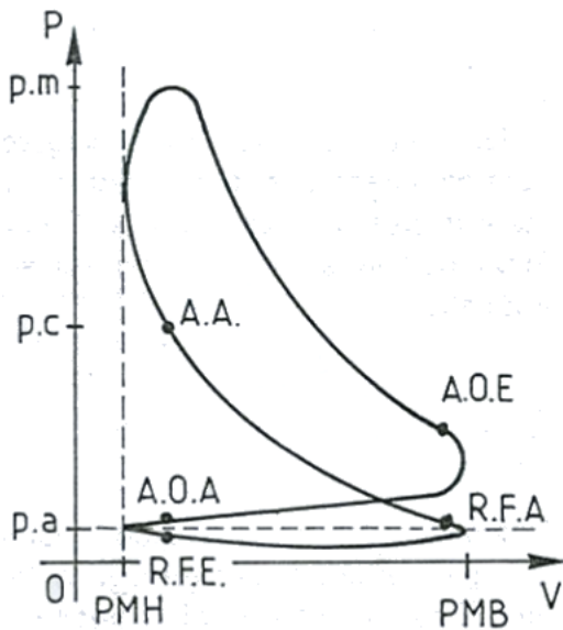
Cycle Beau de Rochas réel (4 temps, essence).
