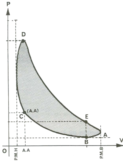
Cycle du moteur à 2 temps.
