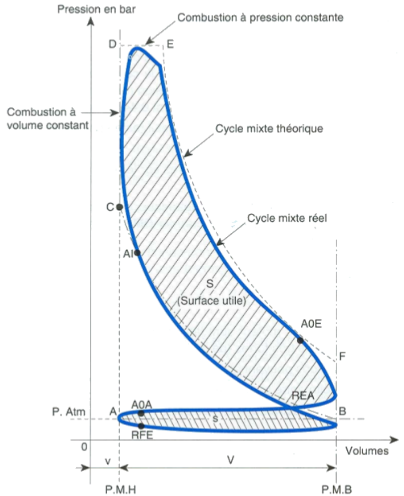
Cycle Diesel mixte réel (4 temps).
