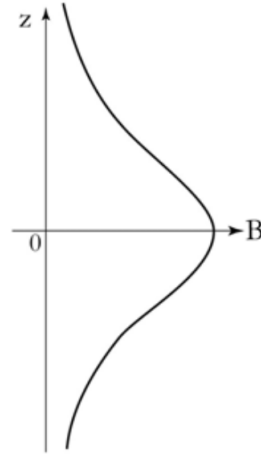
Norme du champ sur l'axe de la spire
