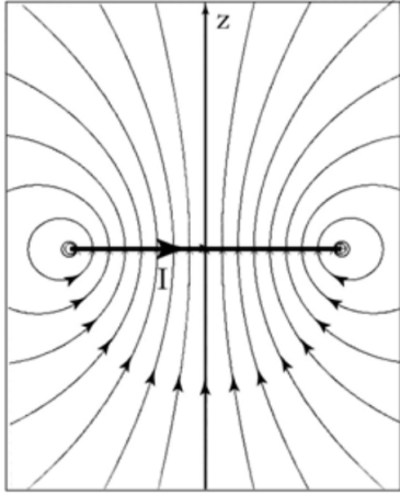
Lignes de champ magnétique
